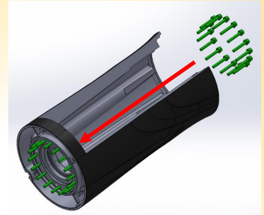
【ボルト挿入例】
